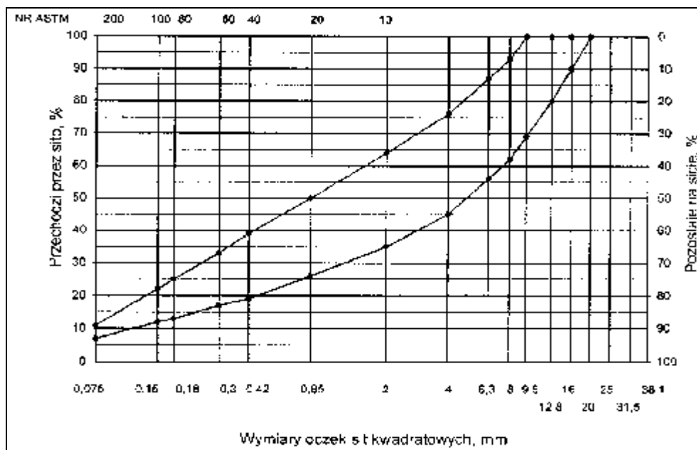
Rys. 1. Krzywe graniczne uziarnienia mieszanki mineralnej BA od 0 do 16mm, od 0 do 12,8 mm do warstwy ścieralnej nawierzchni boisk
