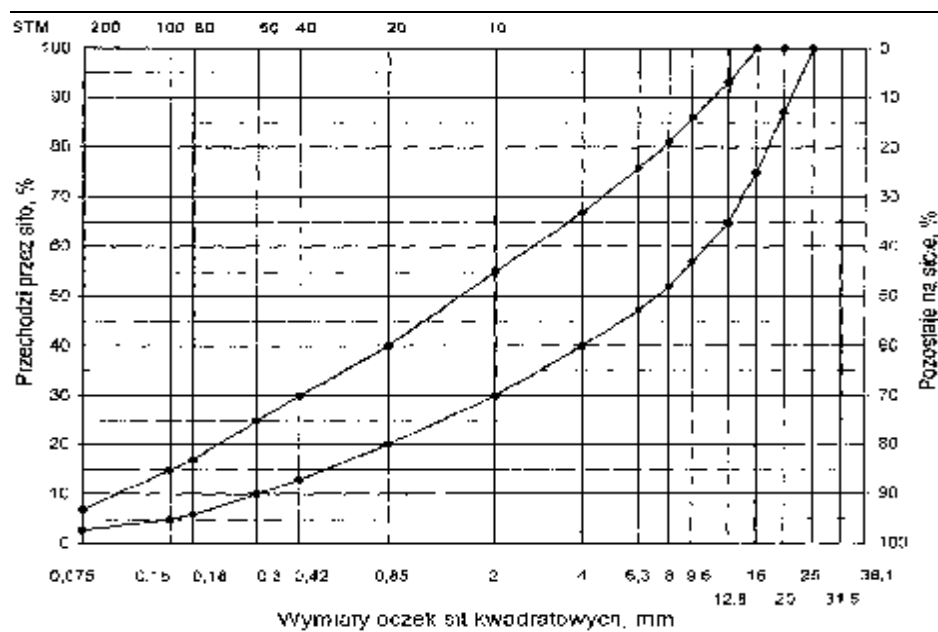
Rys. 2. Krzywe graniczne uziarnienia mieszanki mineralnej BA od 0 do 20 mm do warstwy wiążącej, wyrównawczej i wzmacniającej nawierzchni boisk.
